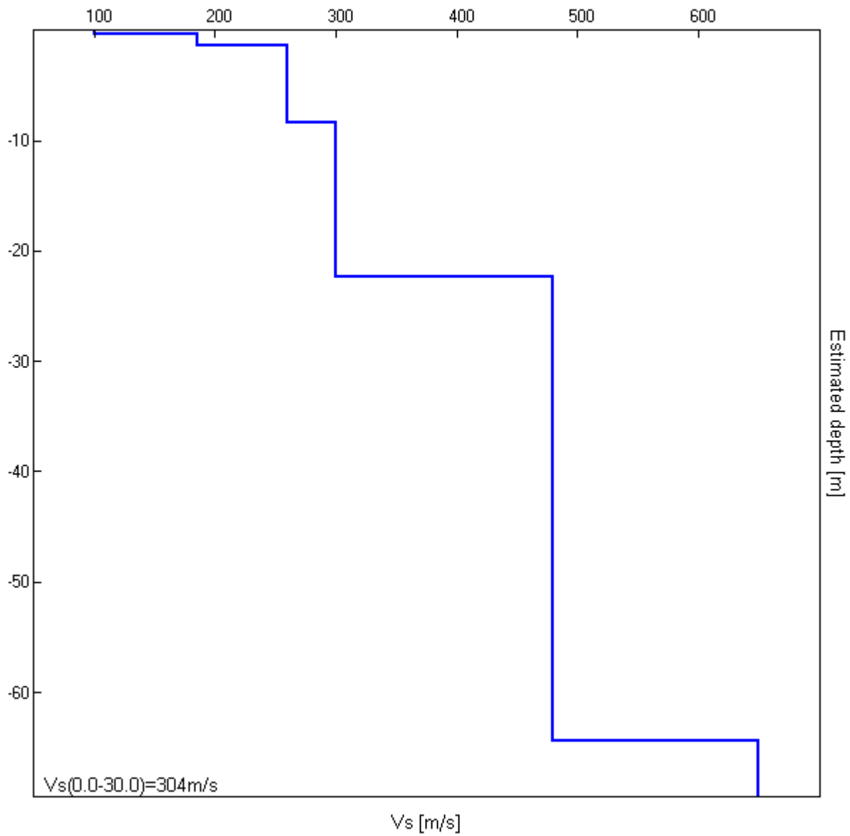
Indagine MASW_5. Profilo verticale delle Vs.
