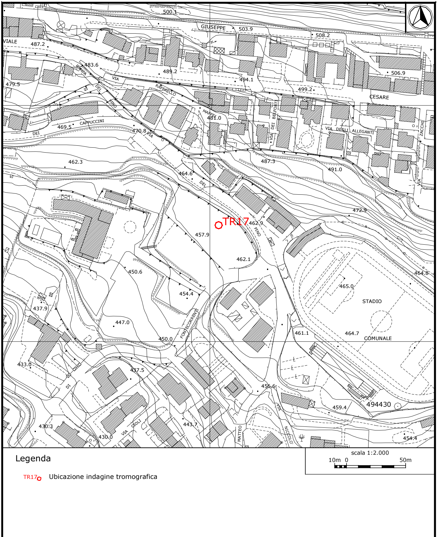
Dettaglio indagine in sismica passiva TR17.
