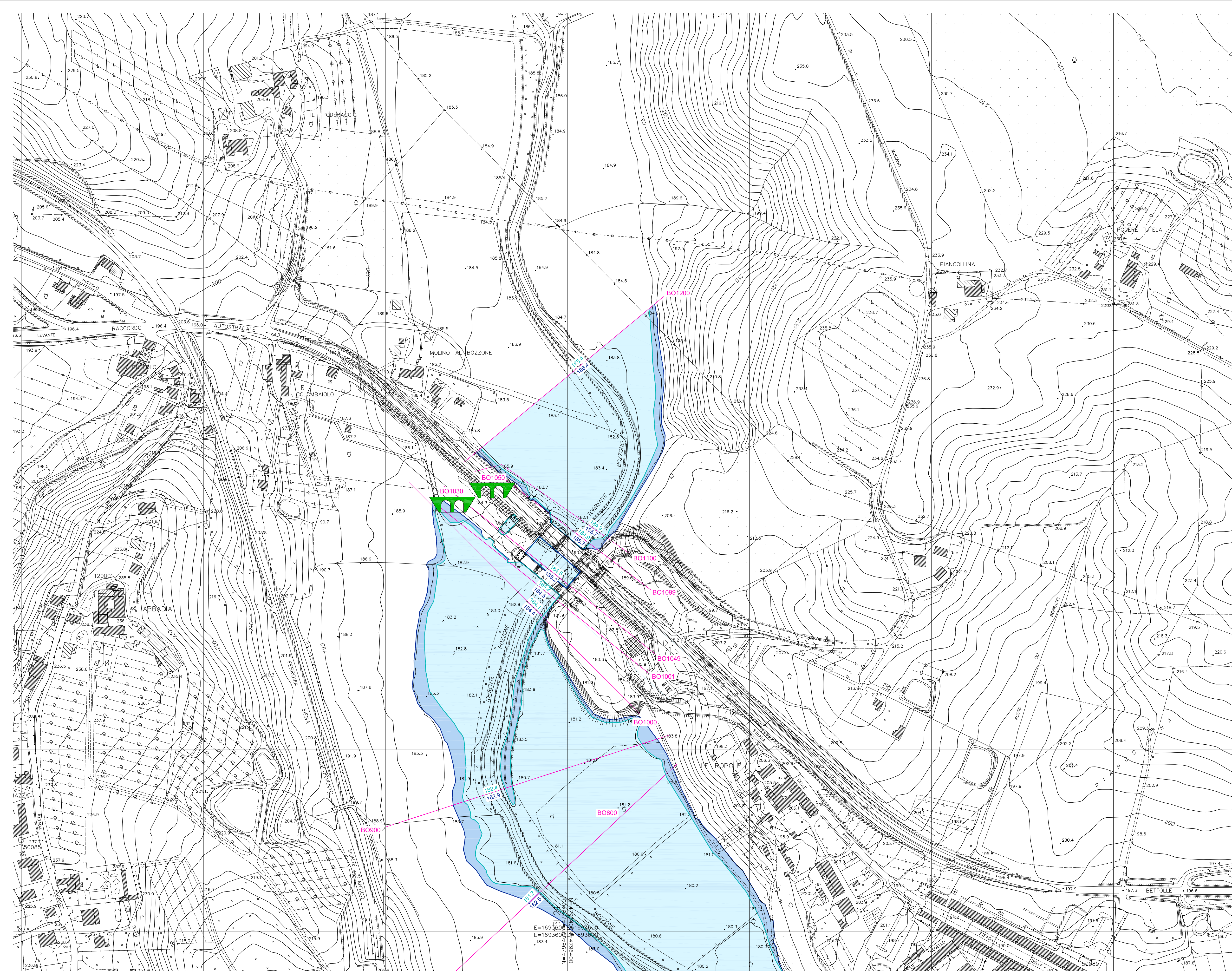
PLANIMETRIE AREE ALLAGATE - T. BOZZONE - INQUADRAMENTO 07.1 (CARTOGRAFIA CTR 1:2000) - 1:2000
