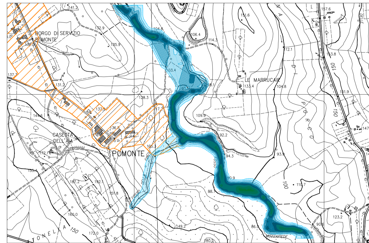
BATTENTI IDRICI EVENTO CON TEMPO DI RITORNO 30 ANNI ABITATO DI POMONTE - Scala 1:10.000
