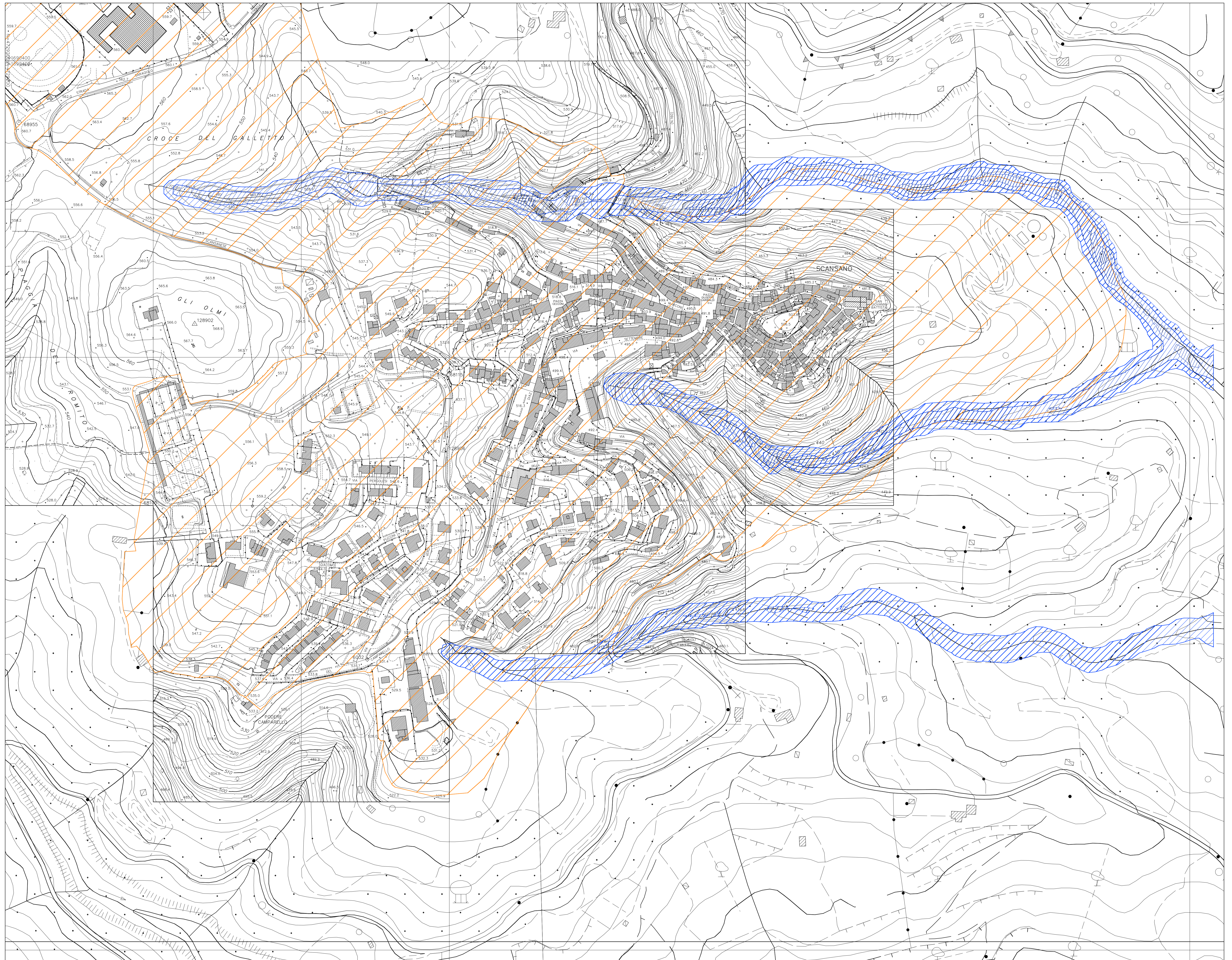
BATTENTI IDRICI EVENTO CON TEMPO DI RITORNO 20 ANNI ABITATO DI SCANSANO - Scala 1:2.000
