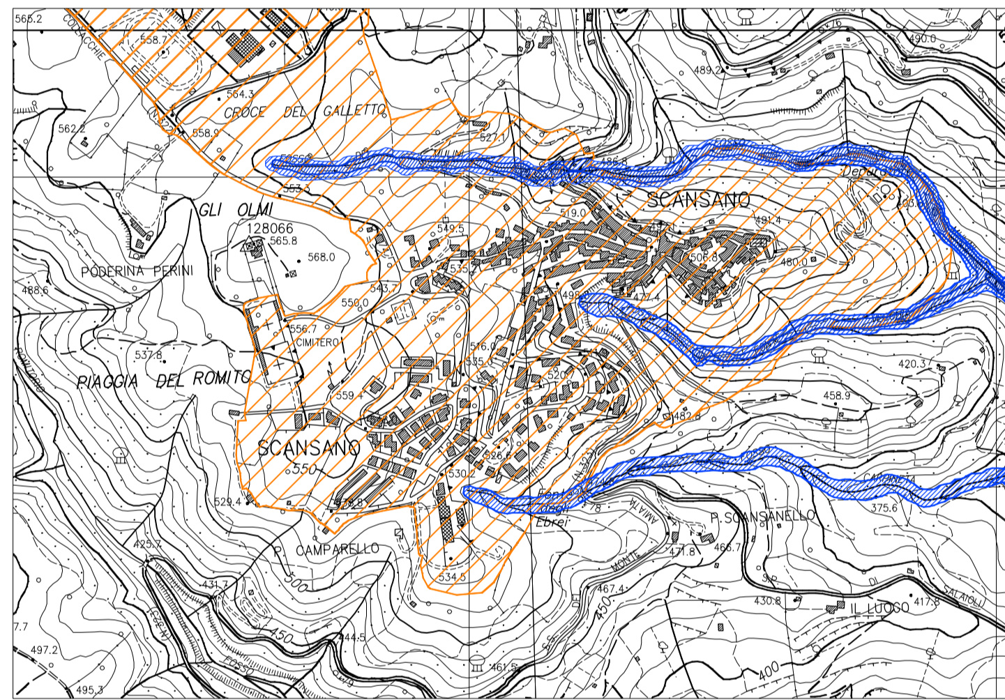
BATTENTI IDRICI EVENTO CON TEMPO DI RITORNO 20 ANNI ABITATO DI SCANSANO - Scala 1:10.000
