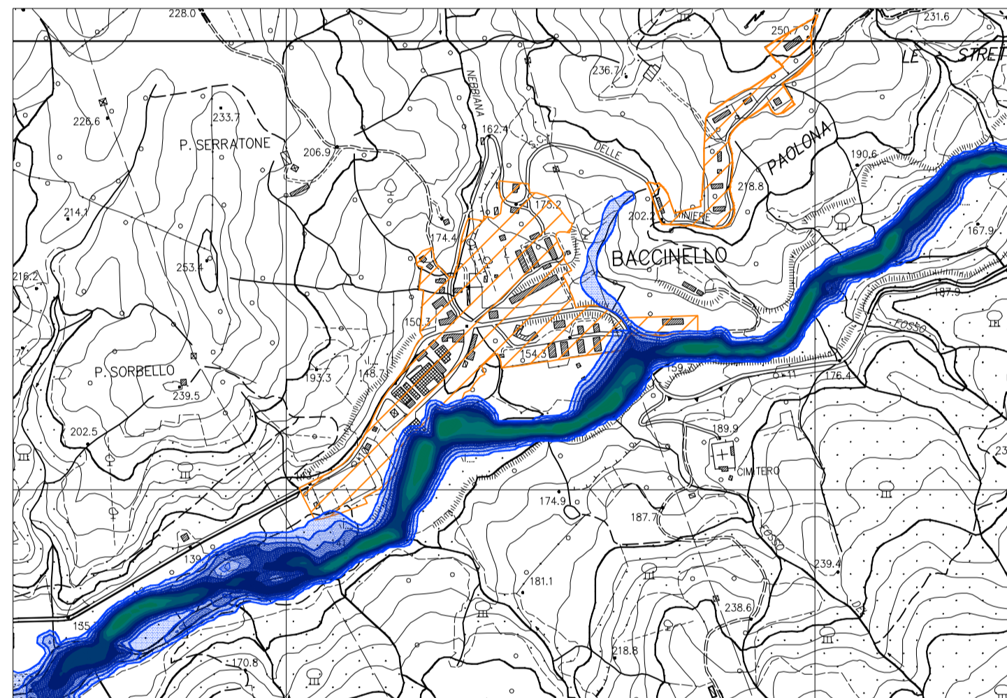
BATTENTI IDRICI EVENTO CON TEMPO DI RITORNO 20 ANNI ABITATO DI BACCINELLO - Scala 1:10.000
