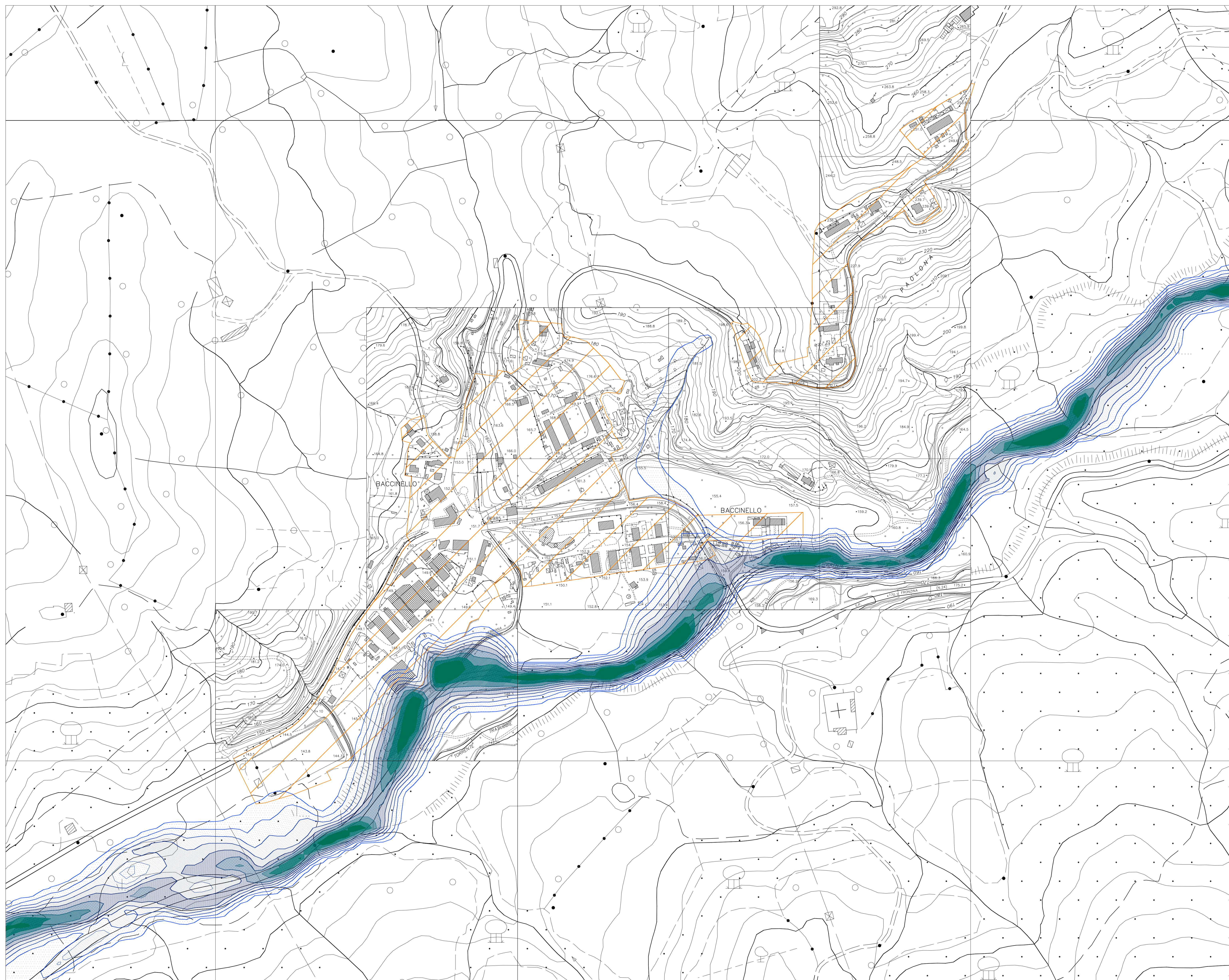
BATTENTI IDRICI EVENTO CON TEMPO DI RITORNO 20 ANNI ABITATO DI BACCINELLO - Scala 1:2.000
