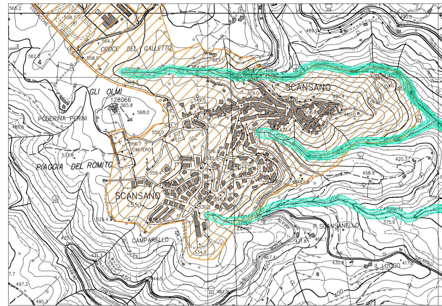
BATTENTI IDRICI EVENTO CON TEMPO DI RITORNO 200 ANNI ABITATO DI SCANSANO - Scala 1:10.000
