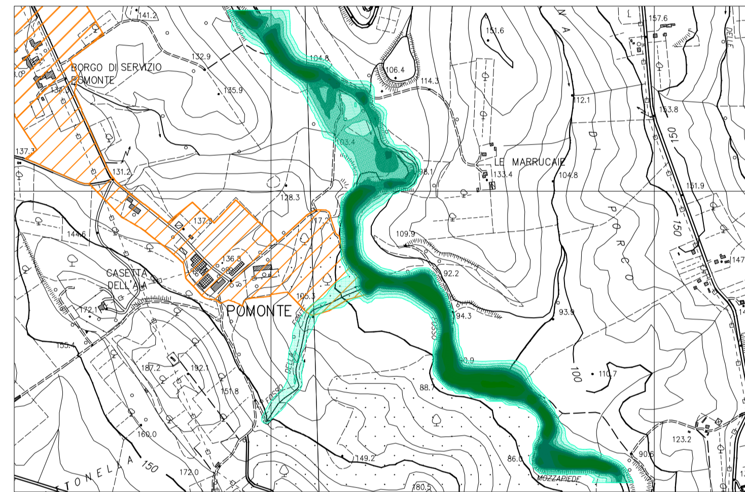
BATTENTI IDRICI EVENTO CON TEMPO DI RITORNO 200 ANNI ABITATO DI POMONTE - Scala 1:10.000
