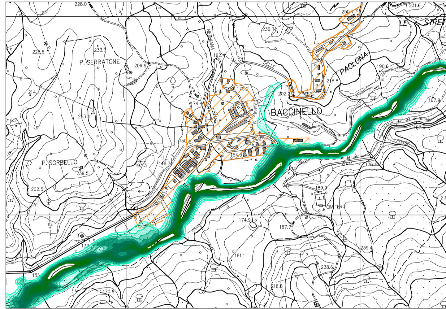
BATTENTI IDRICI EVENTO CON TEMPO DI RITORNO 200 ANNI ABITATO DI BACCINELLO - Scala 1:10.000
