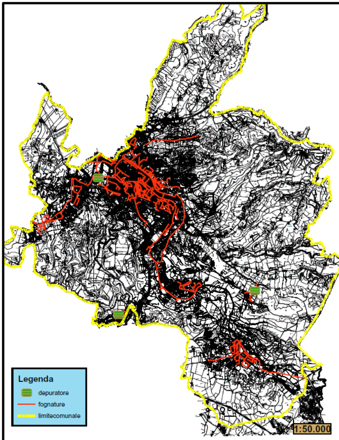
Figura 10. ubicazione impianti di depurazione e rete fognaria
