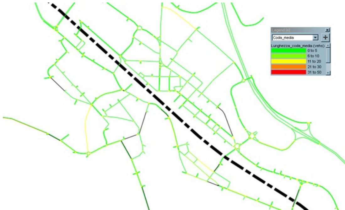
Figura 17: Lunghezza della coda media (numero di veicoli) per l'ora di punta pomeridiana – scenario di progetto
