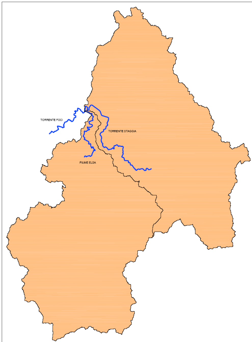
Fig. 20 – Bacino del Fiume Elsa e sottobacino Torrente Staggia alla sezione di confluenza con T. Foci
