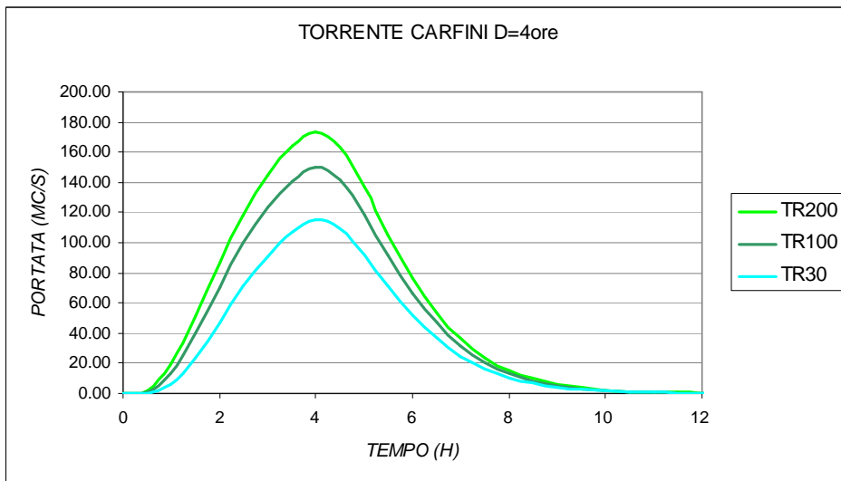
Fig. 25 – Idrogrammi Torrente Carfini introdotti nel modello idraulico per i 3 tempi di ritorno
