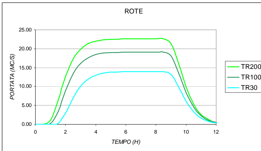
Fig. 17 – Idrogrammi Botro delle Rote per i tempi di ritorno considerati
