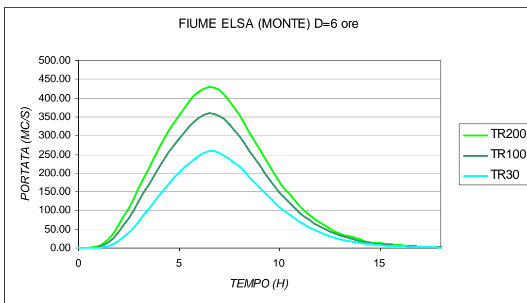
Fig. 21 – Idrogrammi Fiume Elsa in ingresso al modello idraulico di monte per i tempi di ritorno considerati
