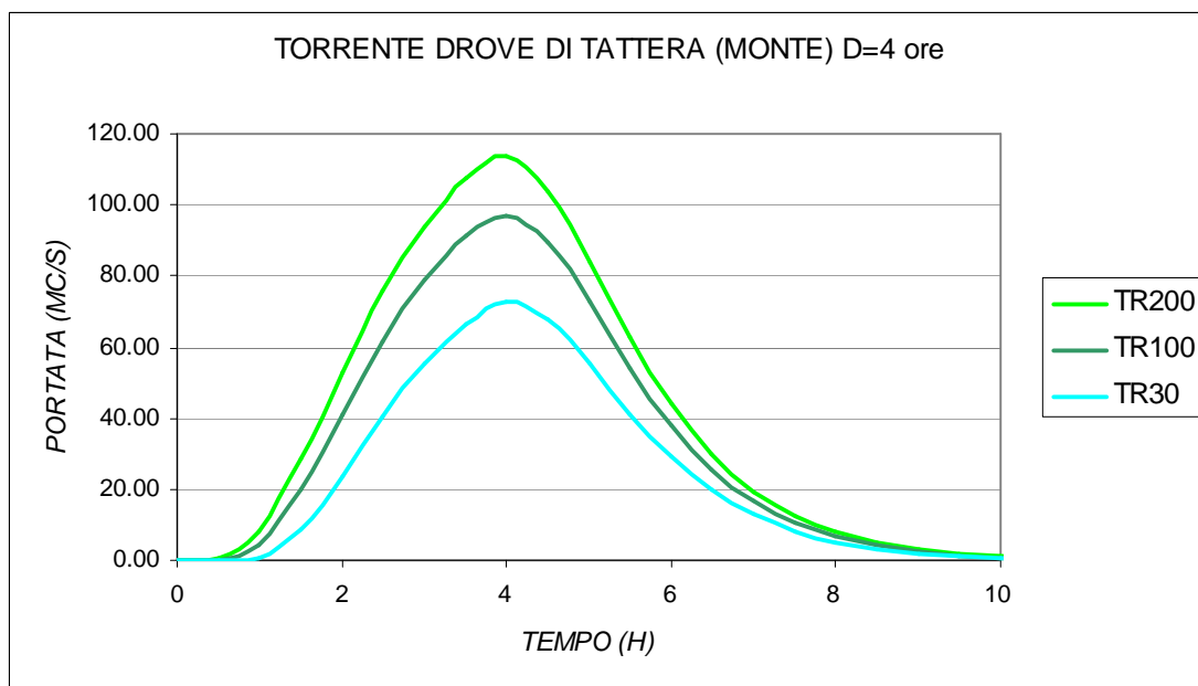
Fig. 34 – Idrogrammi Torrente Drove di Tattera in ingresso al modello idraulico per i 3 tempi di ritorno
