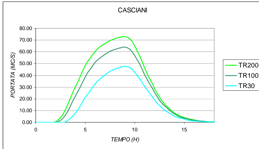
Fig. 19 – Idrogrammi Torrente Casciani per i tempi di ritorno considerati
