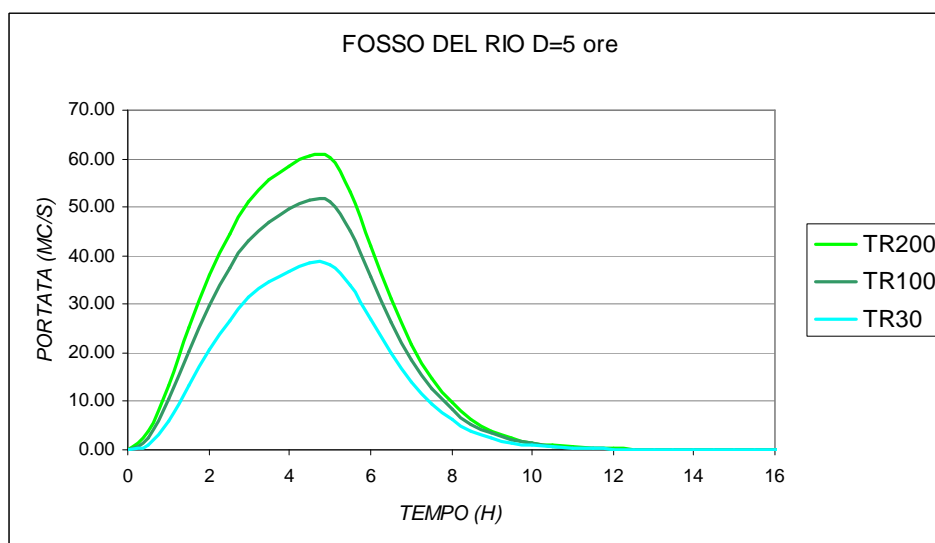
Fig. 32 – Idrogrammi Fosso del Rio introdotti nel modello idraulico per i 3 tempi di ritorno
