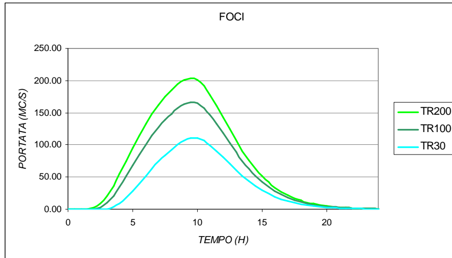
Fig. 10 – Idrogrammi Torrente Foci per i tempi di ritorno considerati
