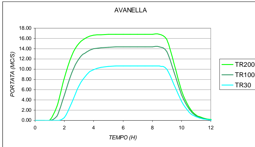
Fig. 16 – Idrogrammi Borro dell'Avanella per i tempi di ritorno considerati
