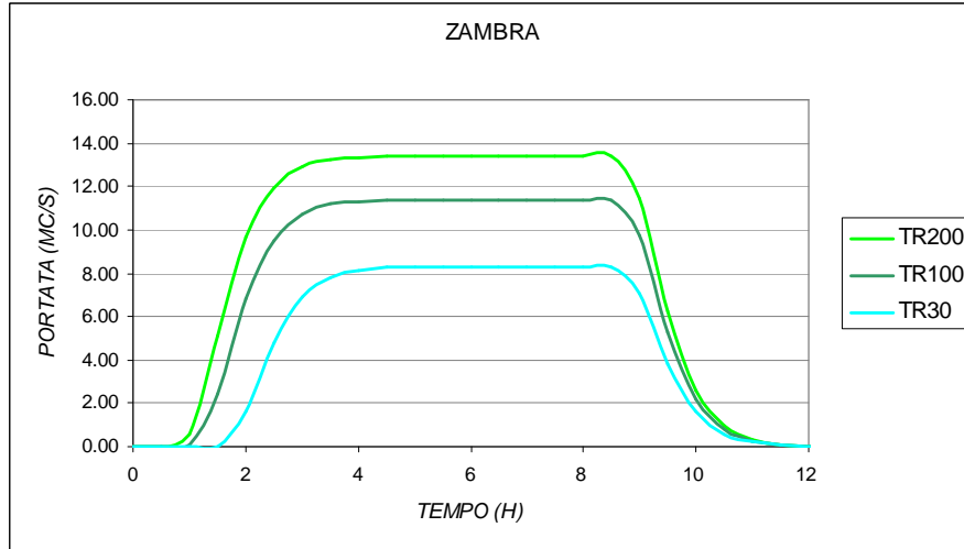
Fig. 13 – Idrogrammi Fosso Zambra per i tempi di ritorno considerati
