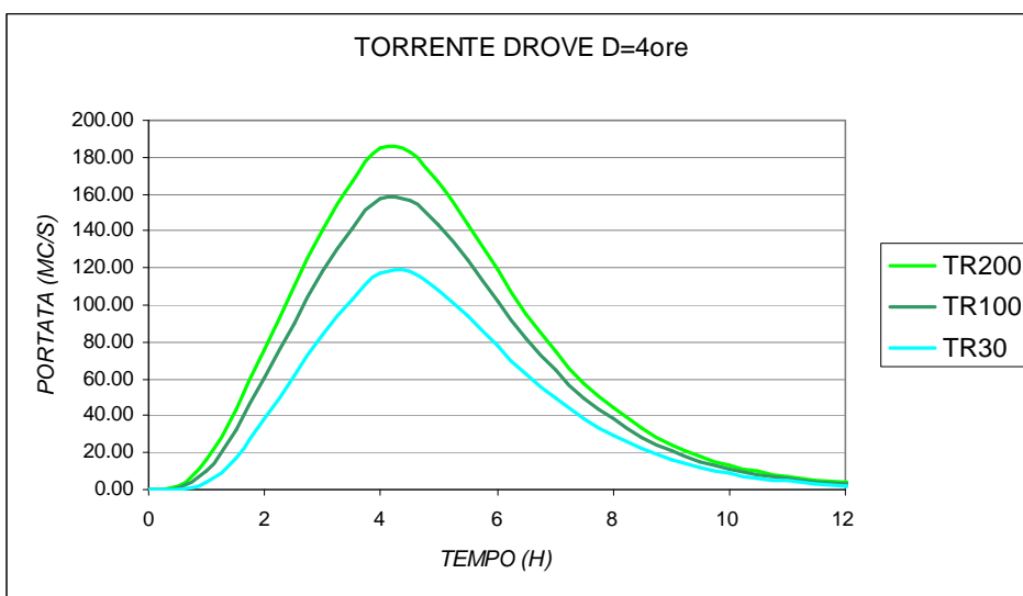
Fig. 29 – Idrogrammi Torrente Drove introdotti nel modello idraulico per i 3 tempi di ritorno
