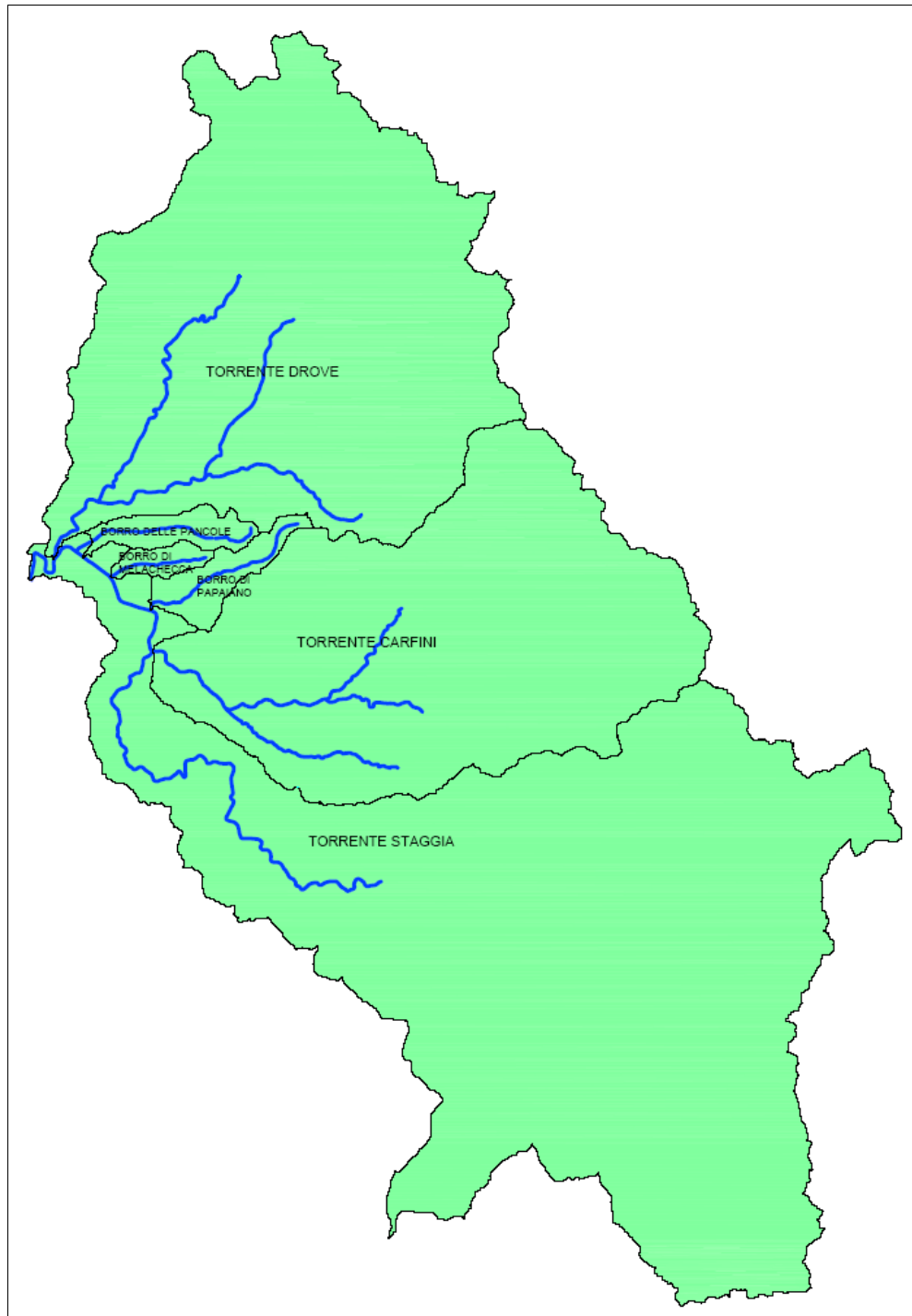
Fig. 23 – Bacino del Torrente Staggia e principali sottobacini alla sezione di confluenza con il Fiume Elsa
