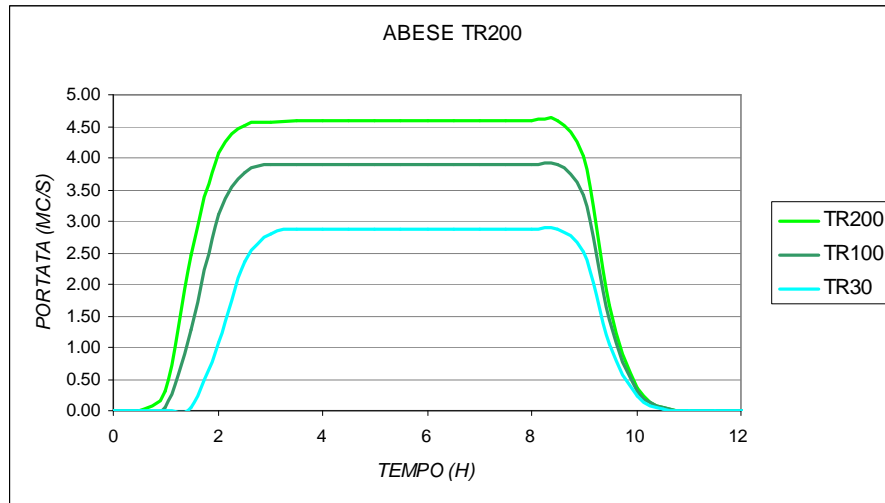
Fig. 11 – Idrogrammi Botro dell'Abese per i tempi di ritorno considerati
