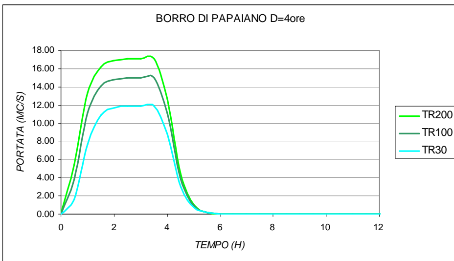
Fig. 26 – Idrogrammi Borro di Papaiano introdotti nel modello idraulico per i 3 tempi di ritorno
