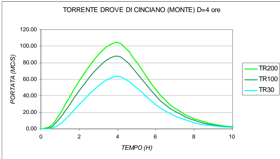
Fig. 35 – Idrogrammi Torrente Drove di Cinciano in ingresso al modello idraulico per i 3 tempi di ritorno
