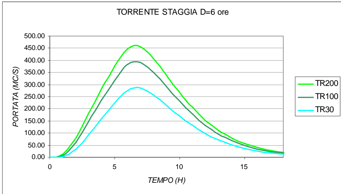
Fig. 22 – Idrogrammi Torrente Staggia introdotti nel modello idraulico per i tempi di ritorno considerati
