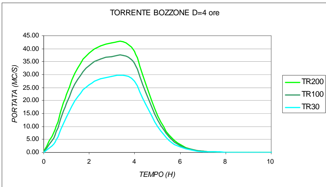
Fig. 36 – Idrogrammi Torrente Bozzone introdotti nel modello idraulico per i 3 tempi di ritorno
