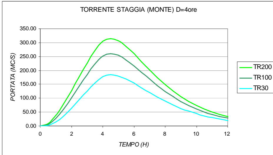
Fig. 24 – Idrogrammi Torrente Staggia in ingresso al modello idraulico di monte per i 3 tempi di ritorno
