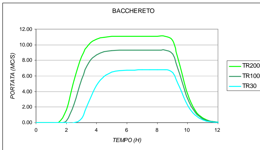
Fig. 12 – Idrogrammi Botro di Bacchereto per i tempi di ritorno considerati
