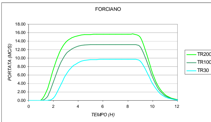
Fig. 15 – Idrogrammi Botro di Forciano per i tempi di ritorno considerati
