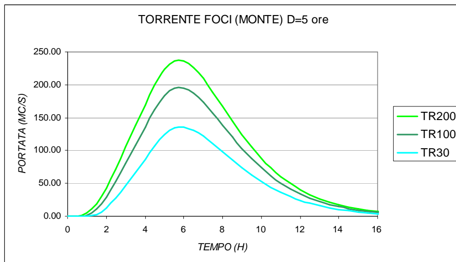
Fig. 31 – Idrogrammi Torrente Foci in ingresso al modello idraulico per i 3 tempi di ritorno
