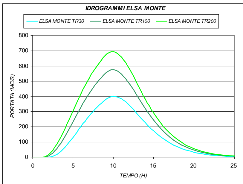
Fig. 9 – Idrogrammi Fiume Elsa in ingresso al modello idraulico per i tempi di ritorno considerati
