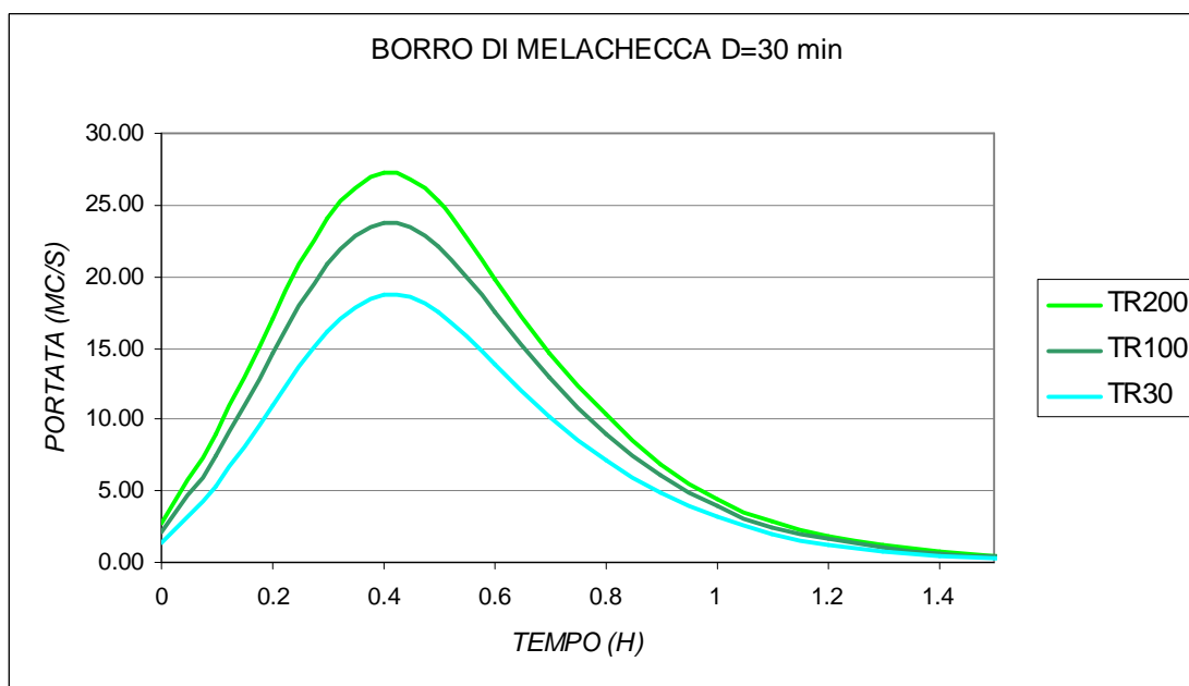
Fig. 38 – Idrogrammi Borro di Melachecca in ingresso al modello idraulico per i 3 tempi di ritorno
