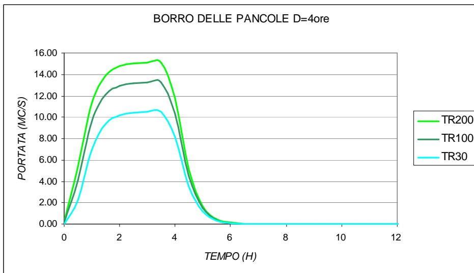
Fig. 28 – Idrogrammi Borro delle Pancole introdotti nel modello idraulico per i 3 tempi di ritorno
