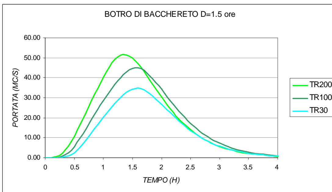
Fig. 37 – Idrogrammi Botro di Bacchereto in ingresso al modello idraulico per i 3 tempi di ritorno
