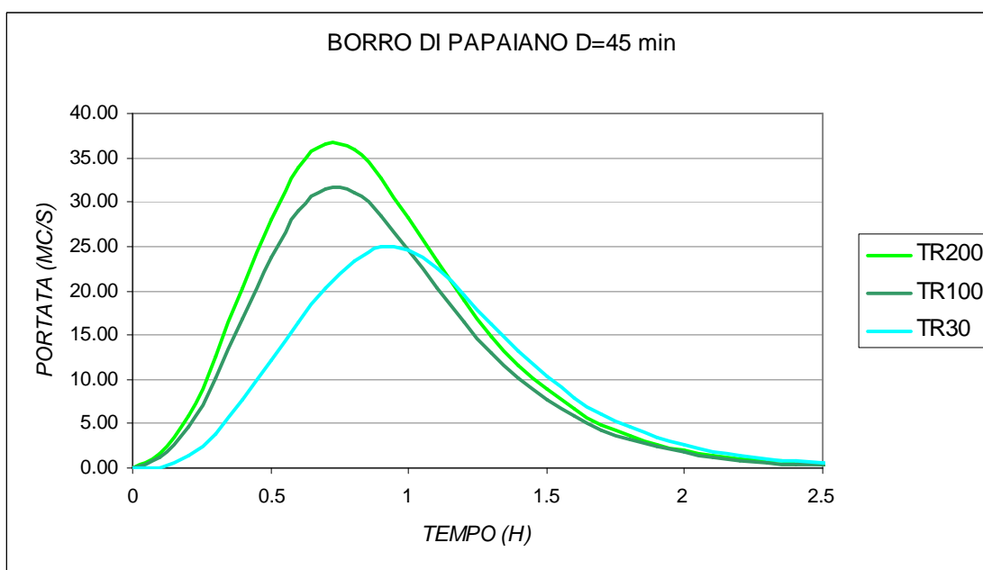
Fig. 39 – Idrogrammi Borro di Papaiano in ingresso al modello idraulico per i 3 tempi di ritorno
