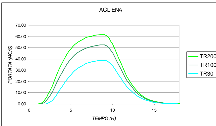
Fig. 18 – Idrogrammi Torrente Agliena per i tempi di ritorno considerati
