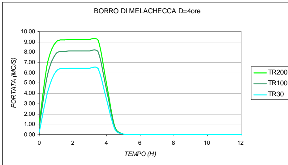
Fig. 27 – Idrogrammi Borro di Melachecca introdotti nel modello idraulico per i 3 tempi di ritorno
