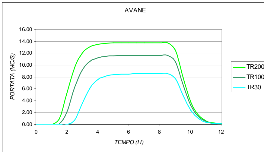
Fig. 14 – Idrogrammi Fosso delle Avane per i tempi di ritorno considerati
