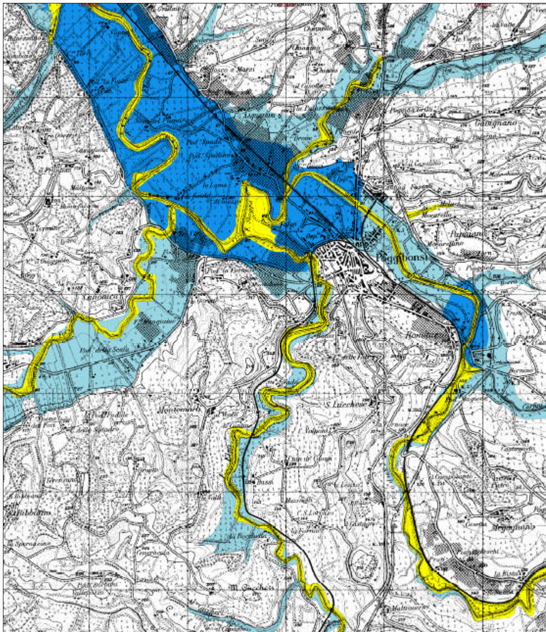
Fig. 7 – Estratto della carta “Perimetrazione delle aree con pericolosità idraulica – Livello di sintesi in scala 1:25.000”, stralcio n. 123, del P.A.I.
