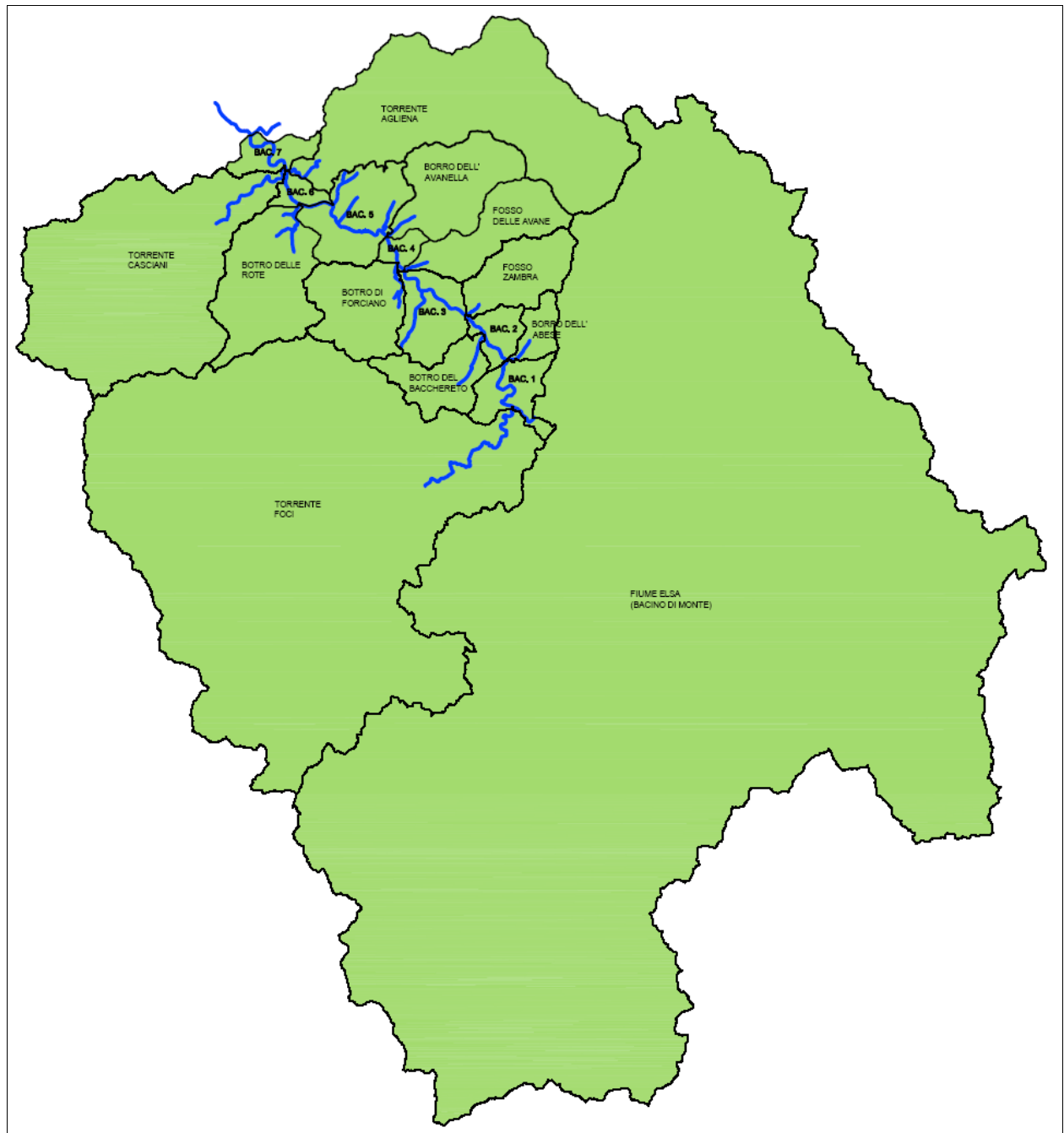
Fig. 8 – Bacino di monte del Fiume Elsa e sottobacini ad esso afferenti nel tratto Poggibonsi – Certaldo
