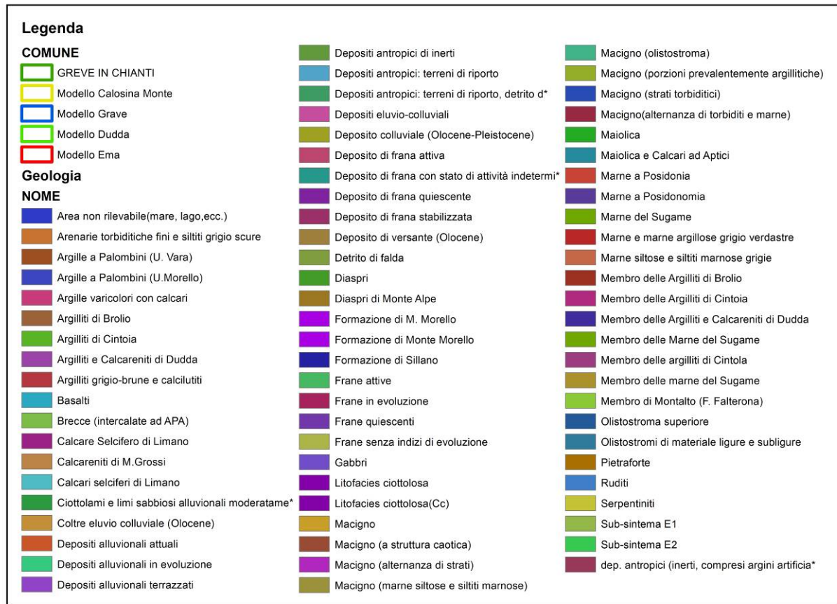
Figura 7 – carta geologica, da cui è stato ricavato il parametro Ks
