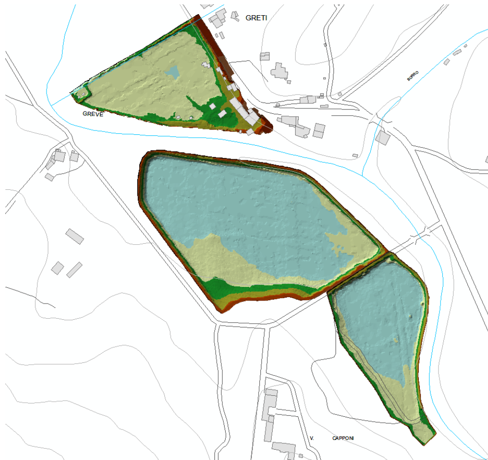
Figura 10 – TIN delle casse di espansione realizzato a partire dal rilievo LIDAR
