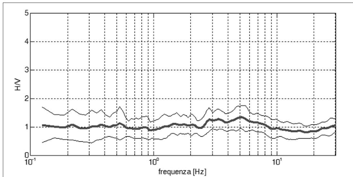
Figura 2 - Curva H/V di un sito su roccia non fratturata e morfologicamente piatta. Si noti l'assenza di amplificazione per risonanza in tutto il dominio delle frequenze.
