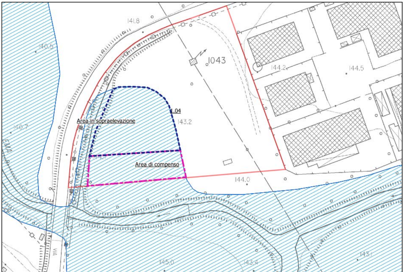
Figura 16 – Interventi di mitigazione del rischio idraulico per l'area d'interesse
