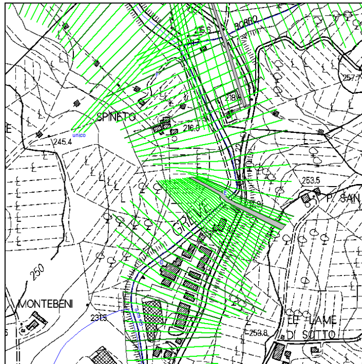
Figura 16 – estratto dalla planimetria del modello idraulico Hec-Ras 4.1.0
