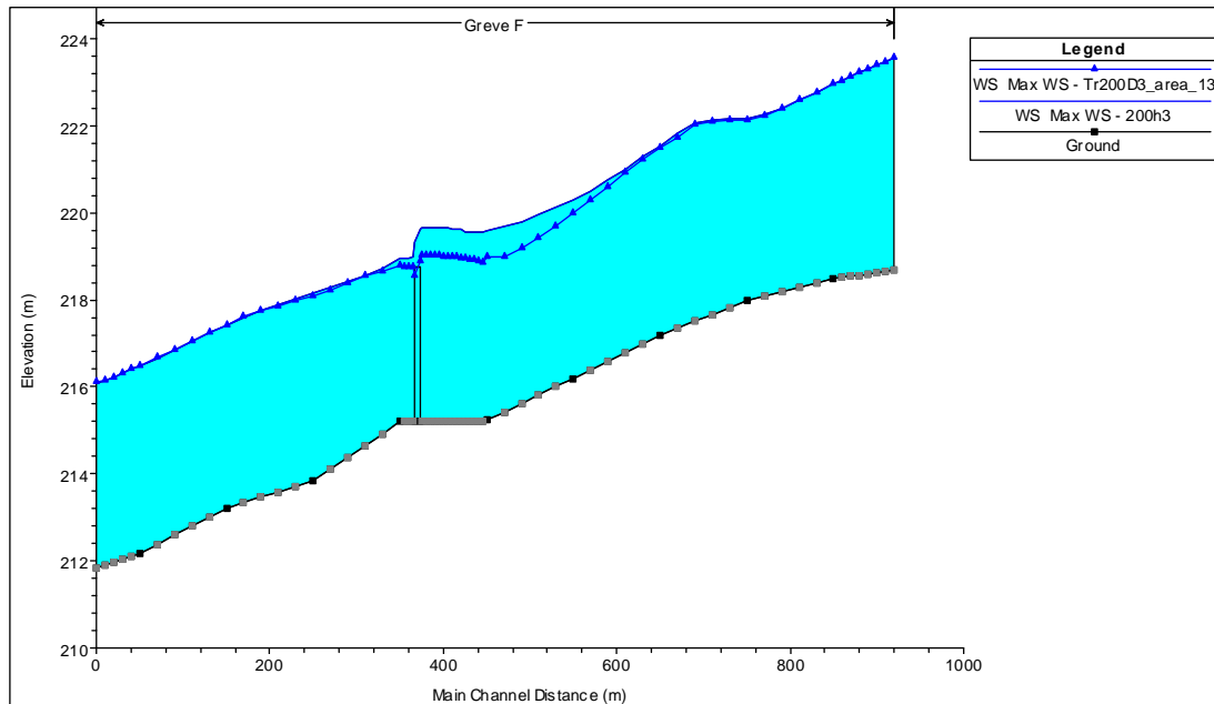
Figura 18 – profilo del Torrente Greve, i due battenti idraulici indicano lo stato attuale (Ws max WS – 200 h3) e lo stato di progetto (Ws max WS – Tr200D3_area_13), l’altezza massima del livello di piena dello stato di progetto non supera il livello dello stato attuale.
