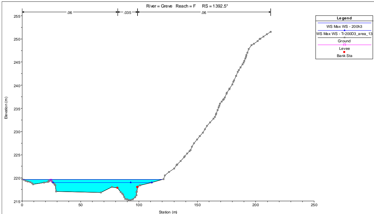
Figura 17 – sezione di progetto immediatamente a monte del ponte sul Torrente Greve, i due battenti idraulici indicano lo stato attuale (Ws max WS – 200 h3) e lo stato di progetto (Ws max WS – Tr200D3_area_13), l'altezza massima del livello di piena dello stato di progetto è contenuta dal rilevato arginale.
