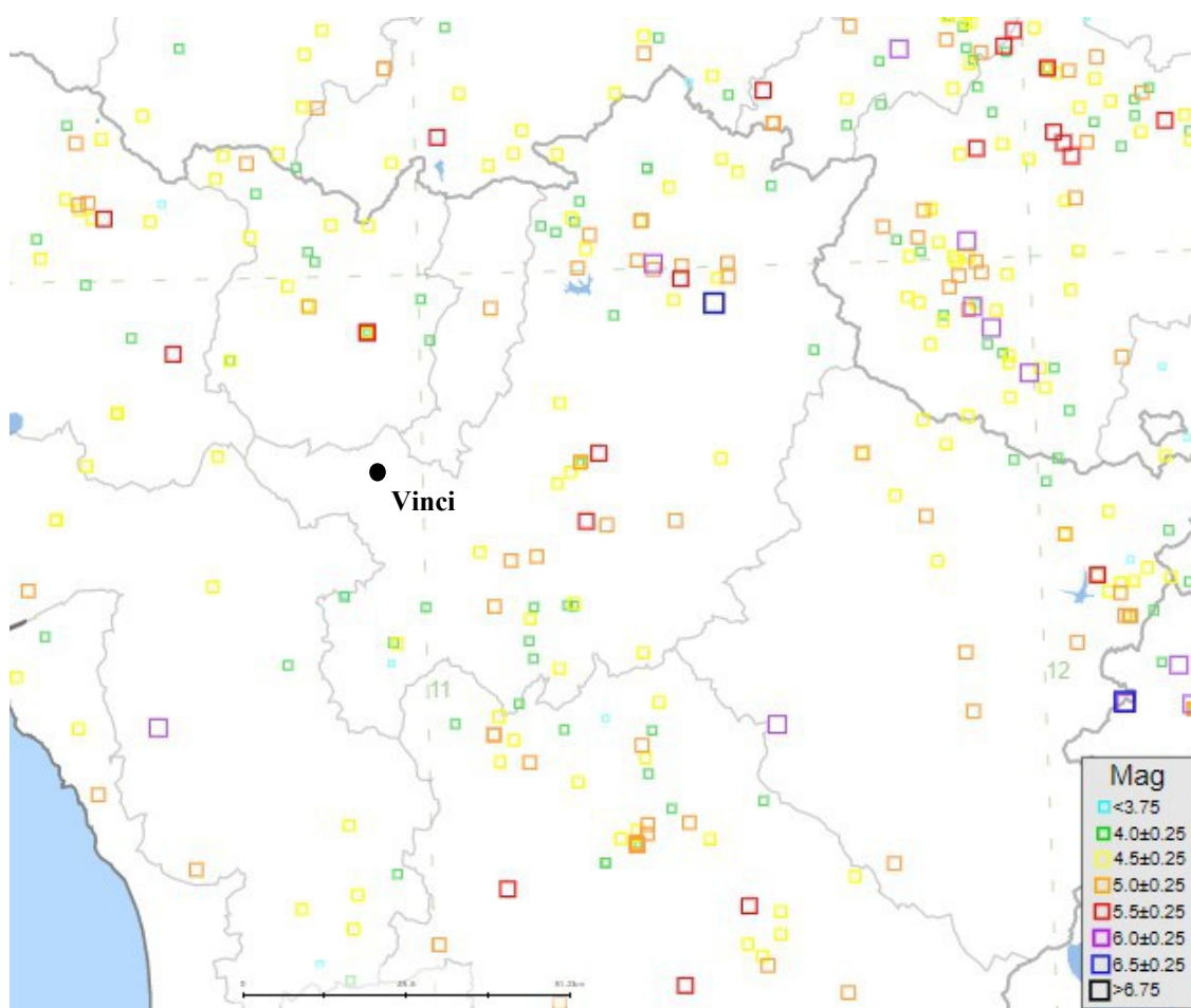
Localizzazione degli eventi macrosismici a livello regionale nel territorio circostante il Comune di Vinci (Periodo 1005 – 2017)
