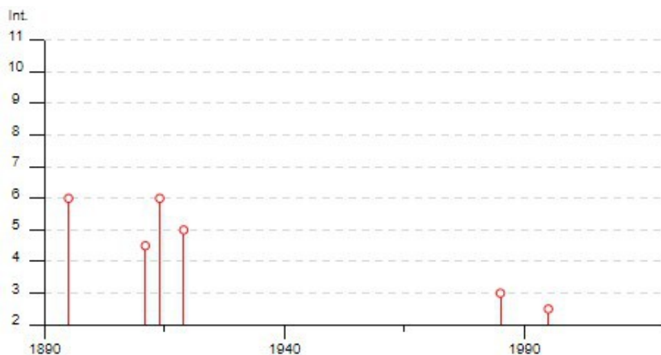
Distribuzione temporale ed intensità degli eventi macrosismici nel periodo 1890-2020
