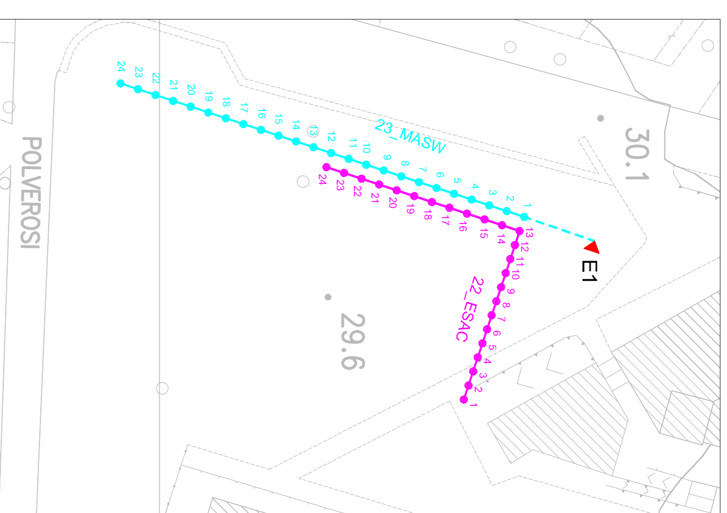
22_ARRAY SISMICO ESAC E 23_MASW - SCALA 1:500
