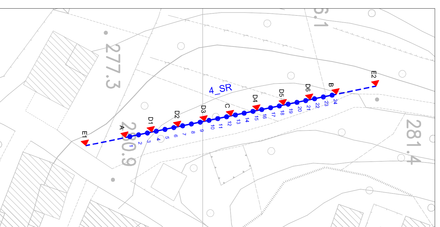
4_SR PROVA SISMICA A RIFRAZIONE ONDE P E ONDE SH - SCALA 1:500
