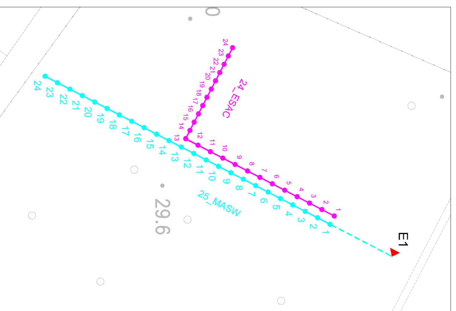
24_ARRAY SISMICO ESAC E 25_MASW - SCALA 1:500
