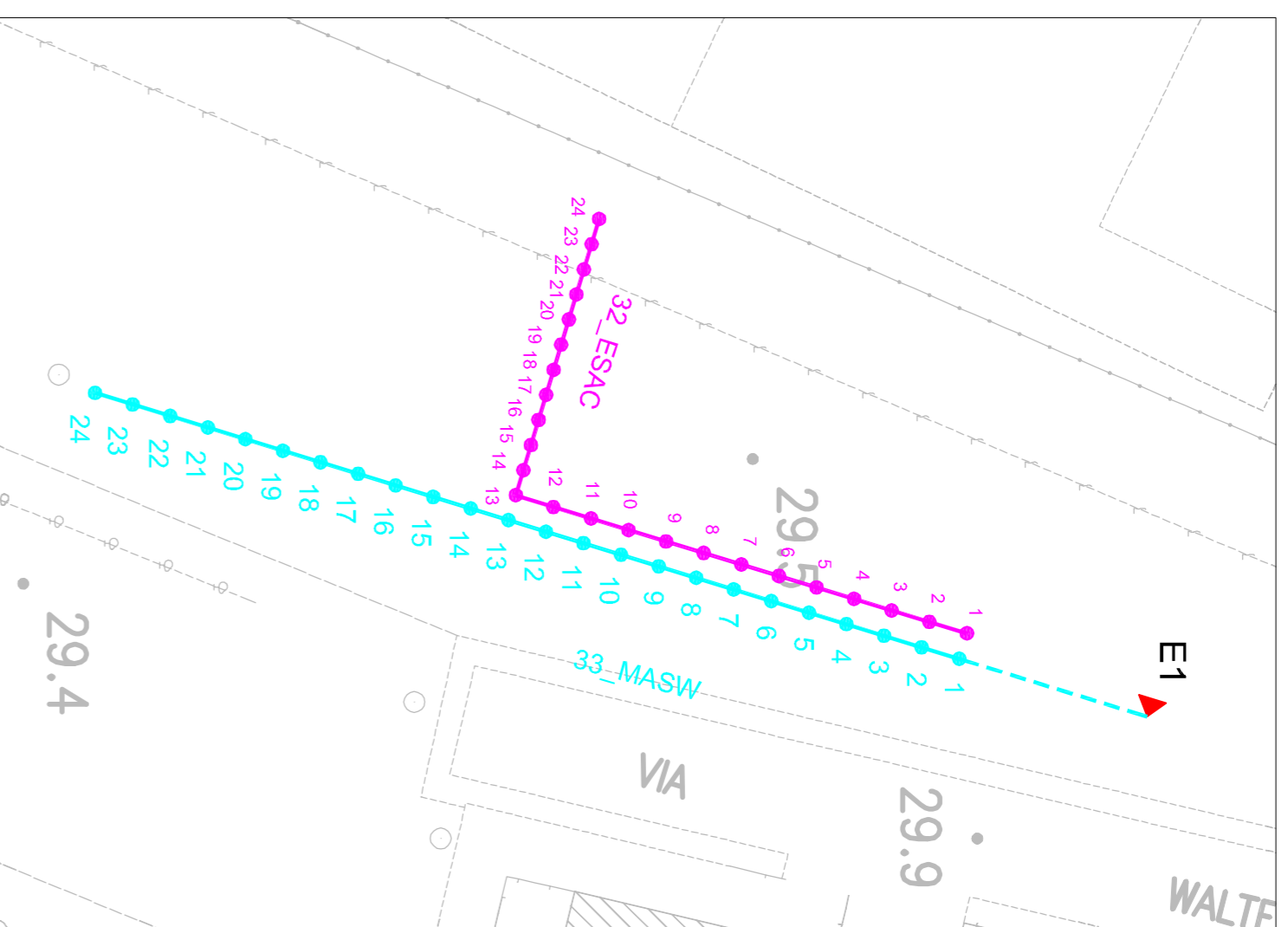
32_ARRAY SISMICO ESAC E 33_MASW - SCALA 1:500
