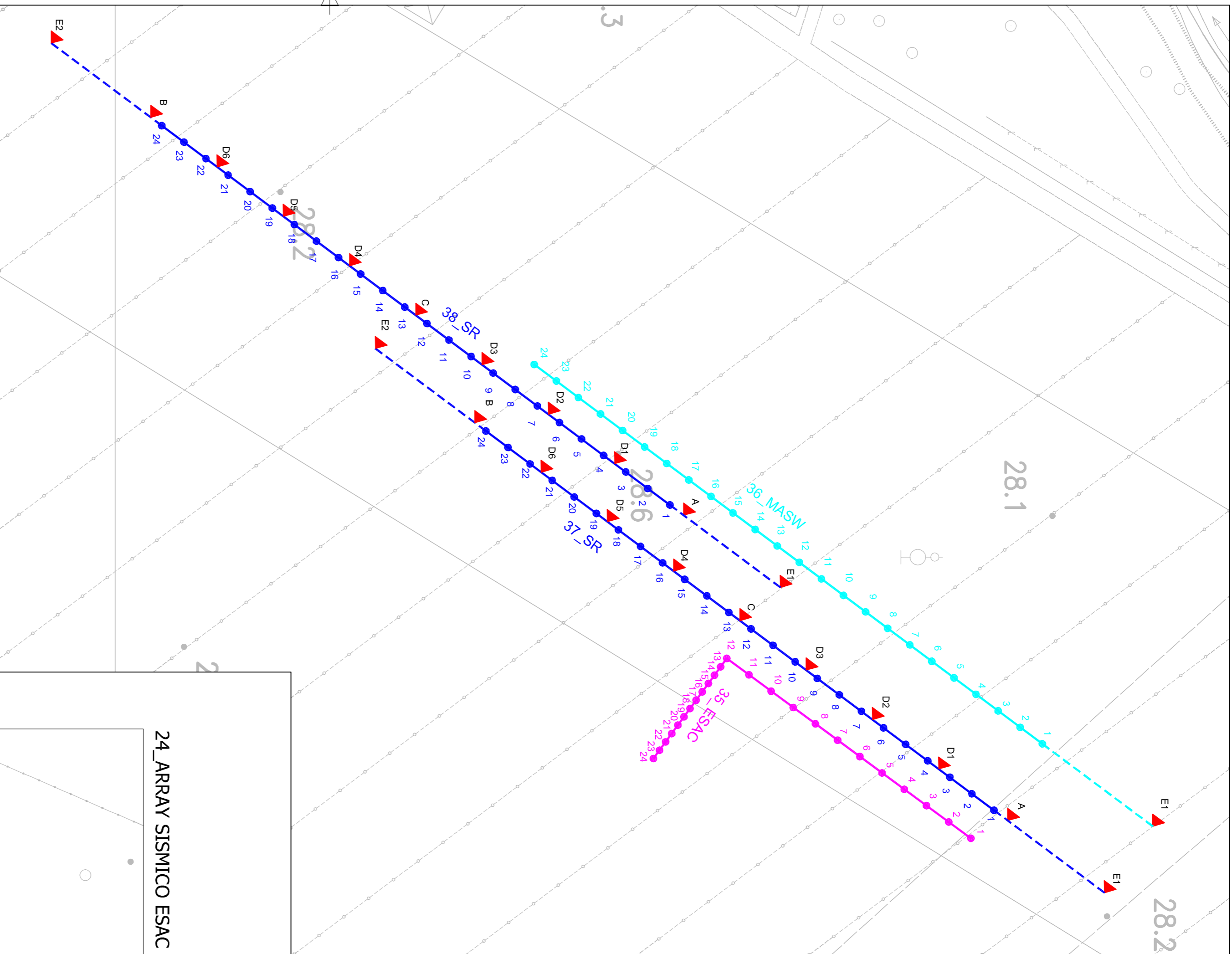
35_ARRAY SISMICO ESAC, 36_MASW, 37-38 PROVE SISMICHE A RIFRAZIONE ONDE P E ONDE SH - SCALA 1:500
