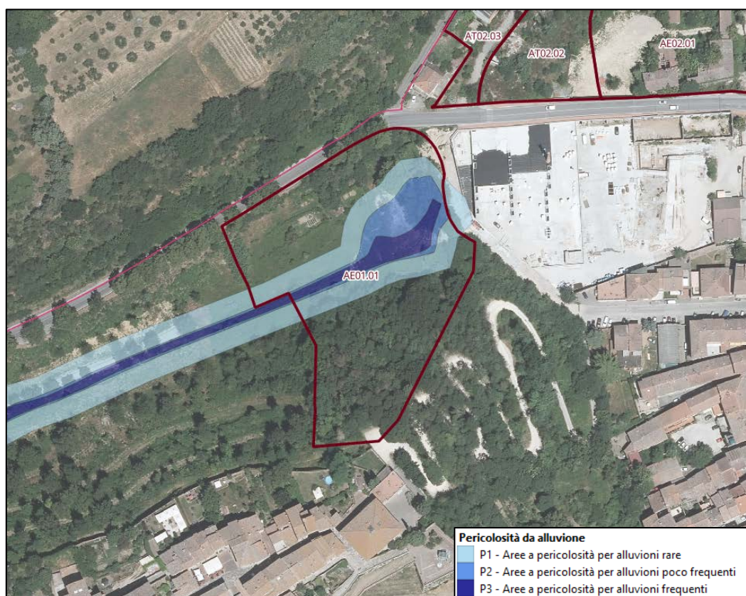
Figura 2.1 – Inquadramento dell'intervento
