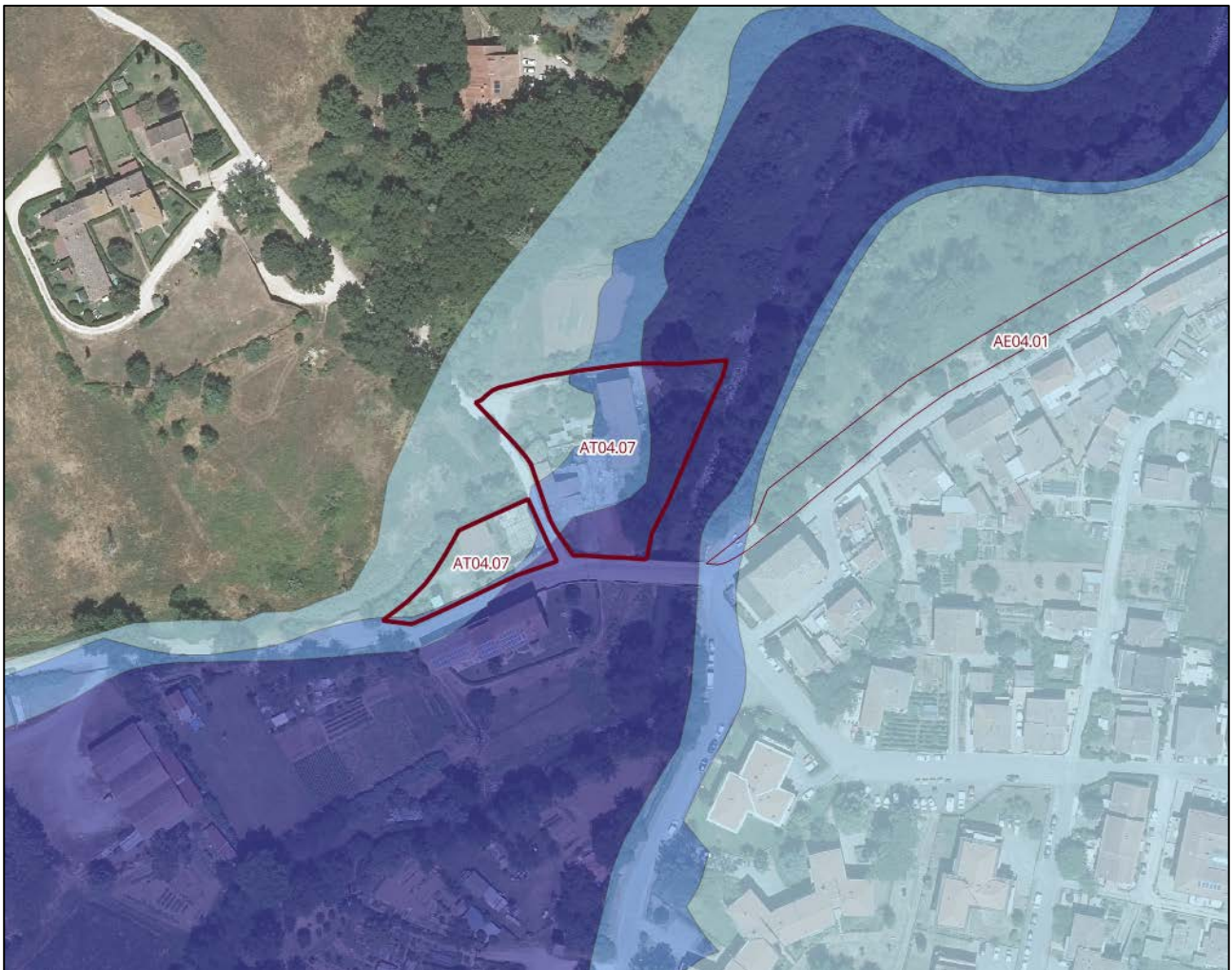
Figura 2.42 – Inquadramento dell'intervento
