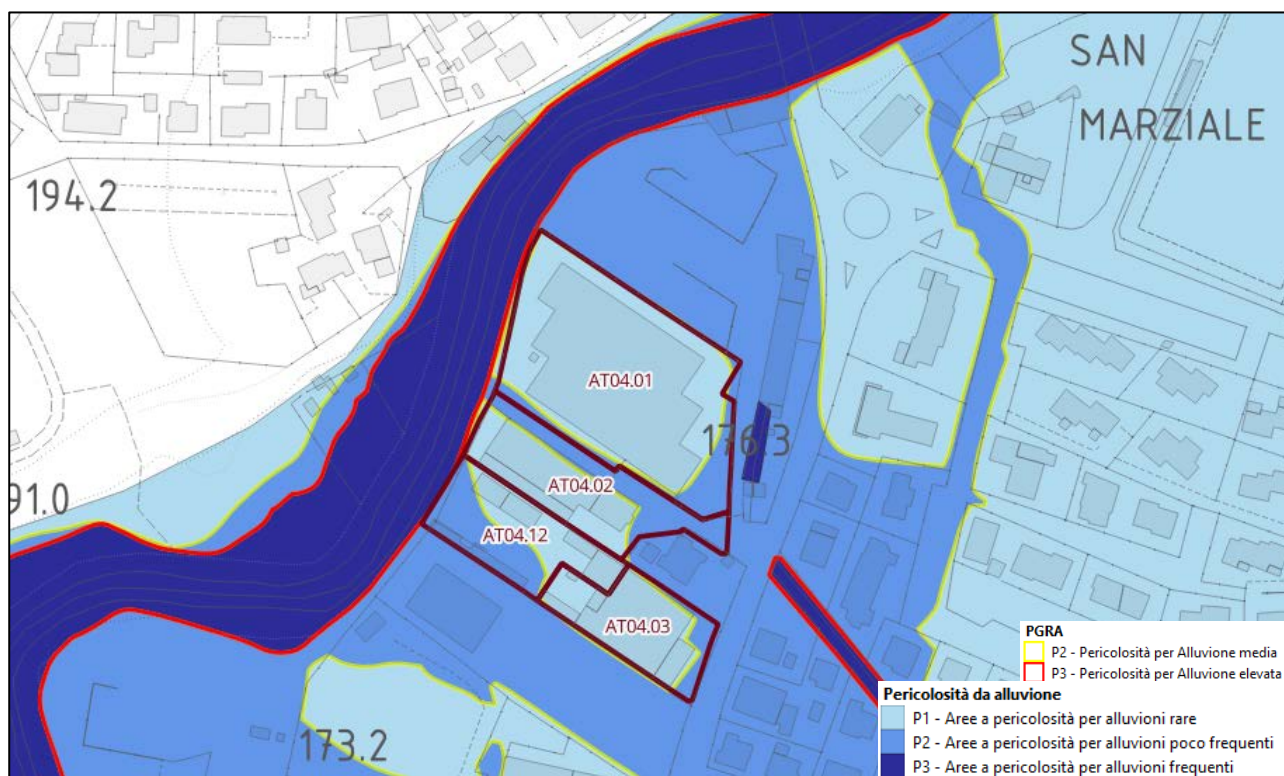
Figura 2.30 – Inquadramento dell'intervento
