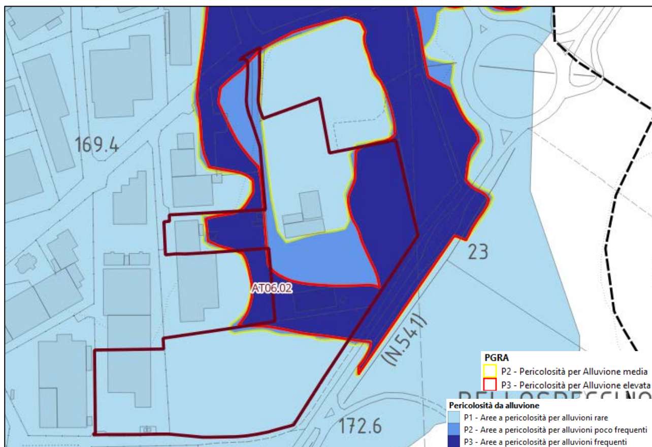
Figura 2.50 – Inquadramento dell'intervento
