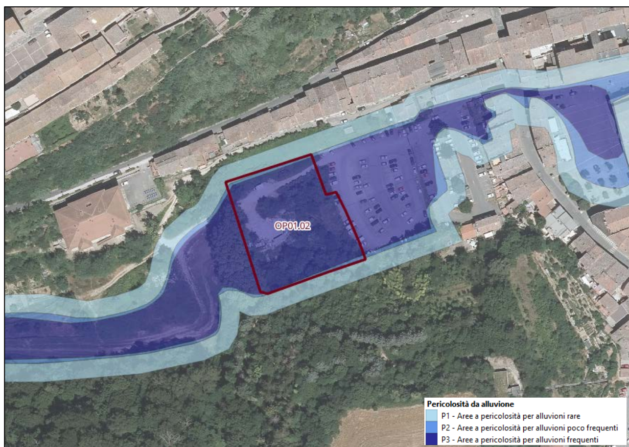
Figura 2.14 – Inquadramento dell'intervento
