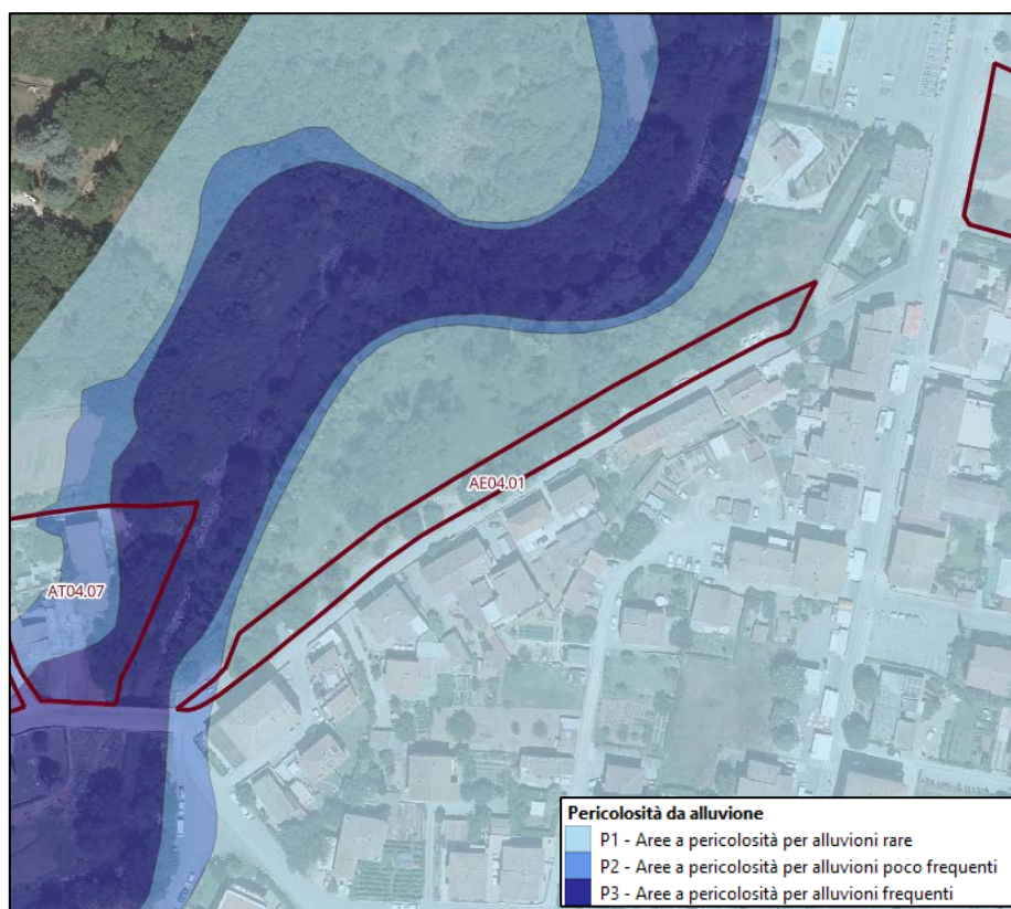
Figura 2.3 – Inquadramento dell'intervento
