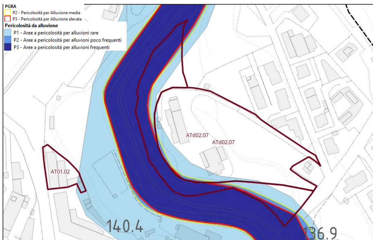
Figura 2.20 – Inquadramento dell'intervento
