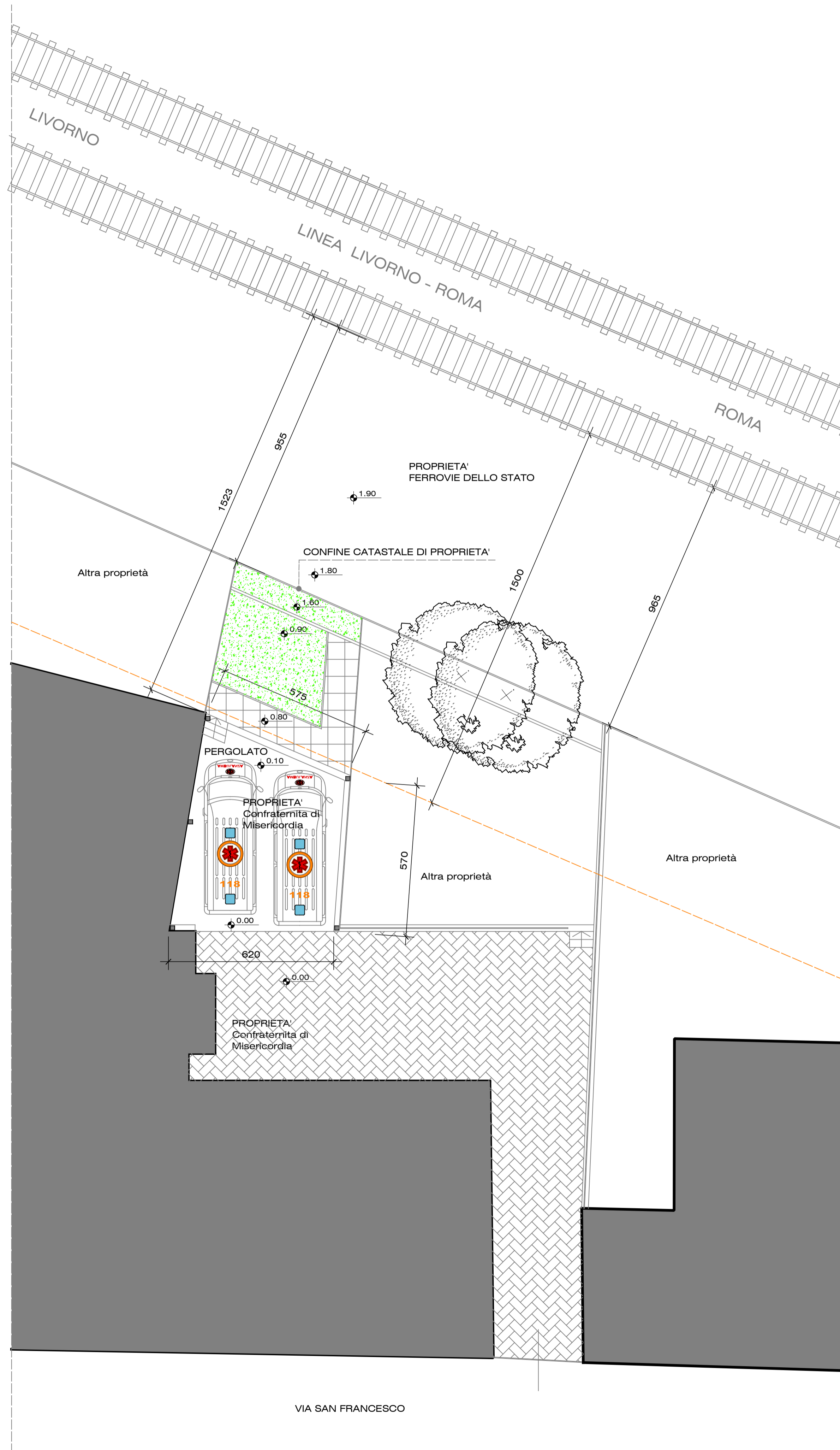
PLANIMETRIA 1:100 MODIFICATO
