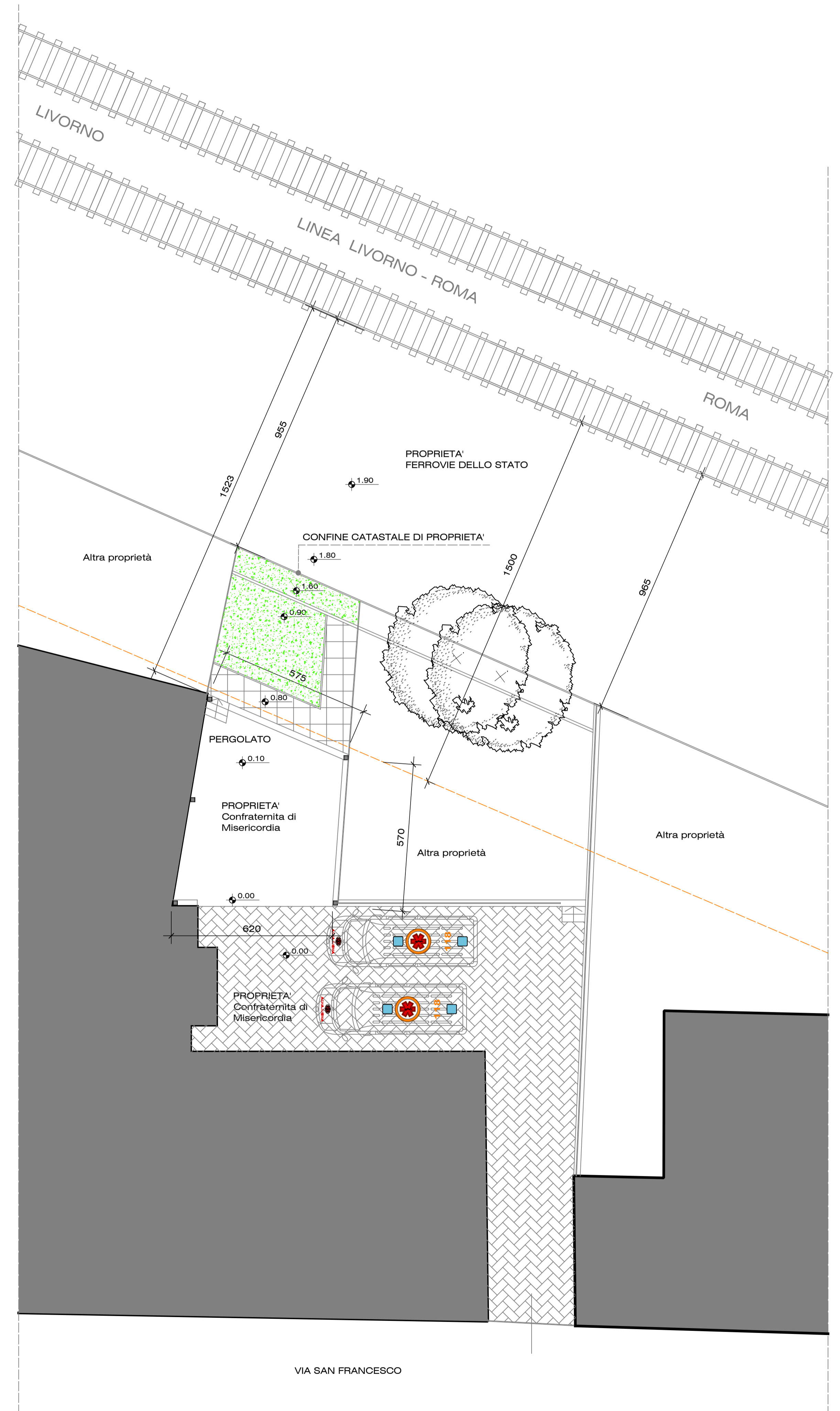
PLANIMETRIA 1:100 MODIFICATO_2
