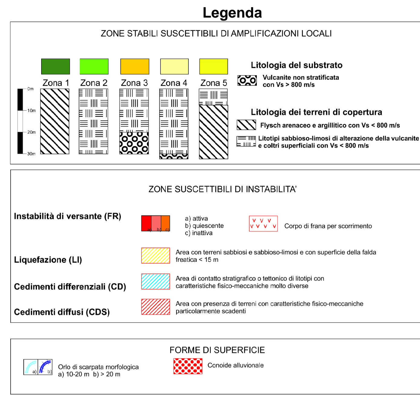
Tav. G1e - Carta delle Microzone Omogenee in Prospettiva Sismica
