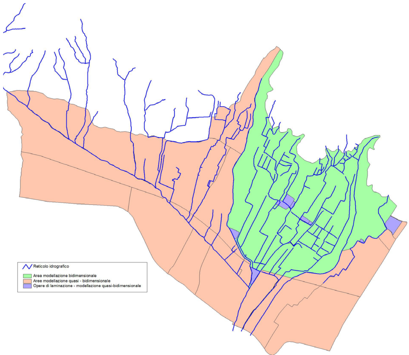
Figura 2-2-Area modellazione quasi - bidimensionale.
