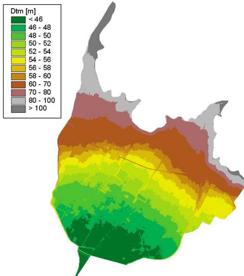
Figura 2-1 -Area modellazione bidimensionale.
