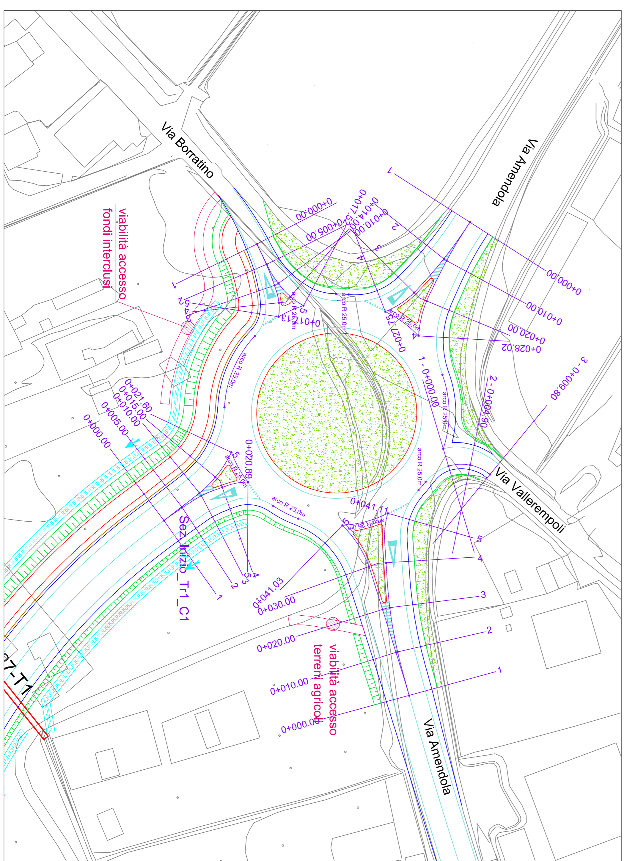
Rami di ingresso/uscita: planimetria di progetto e tracciamento sezioni
